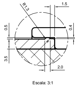
Detalle B
