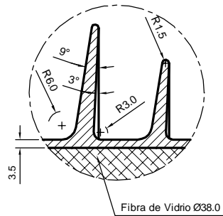
Detalle A
